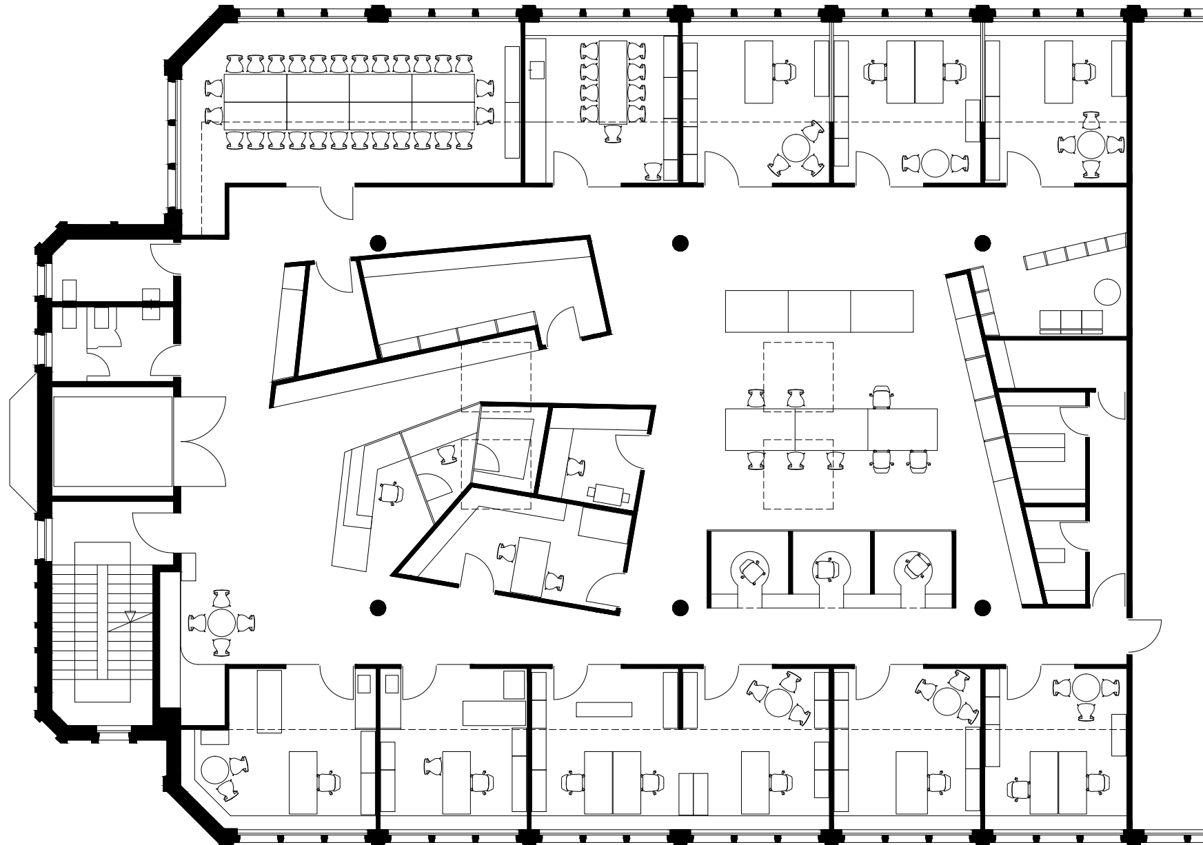
GRUNDRISS
