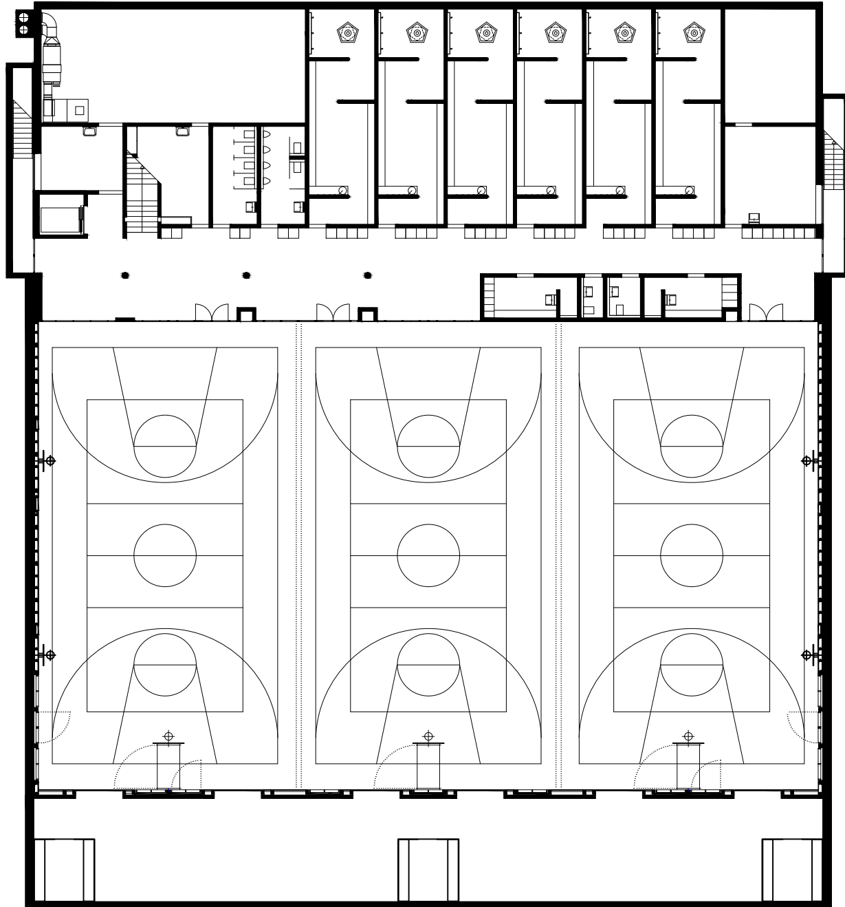
GRUNDRISS UG 0 5 10 15 20
